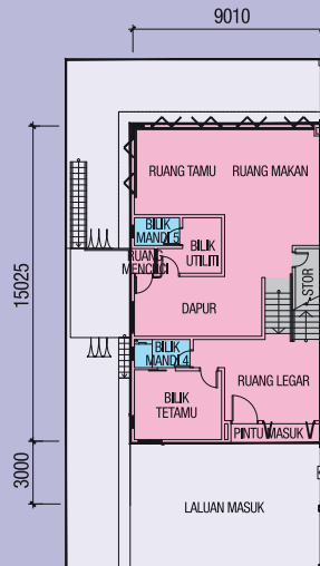
PELAN LANTAI TINGKAT BAWAH
